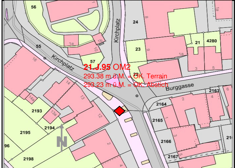
Situationsplan MuttENZ
